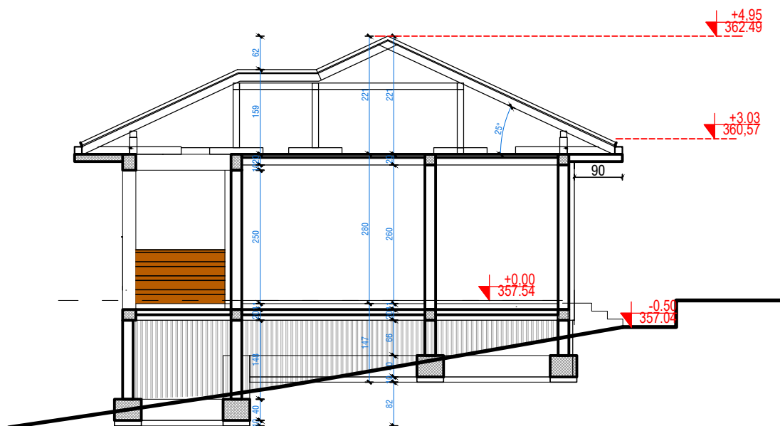
PRESEK 2-2
