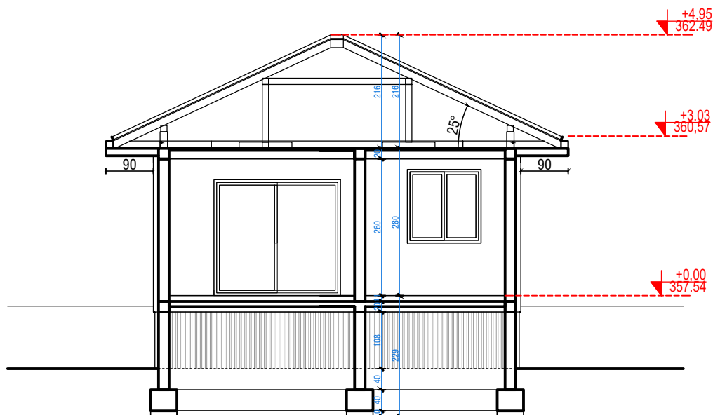
PRESEK 1-1
